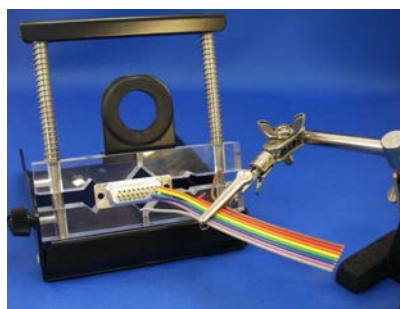
治具「てだすけ君」を使った固定
